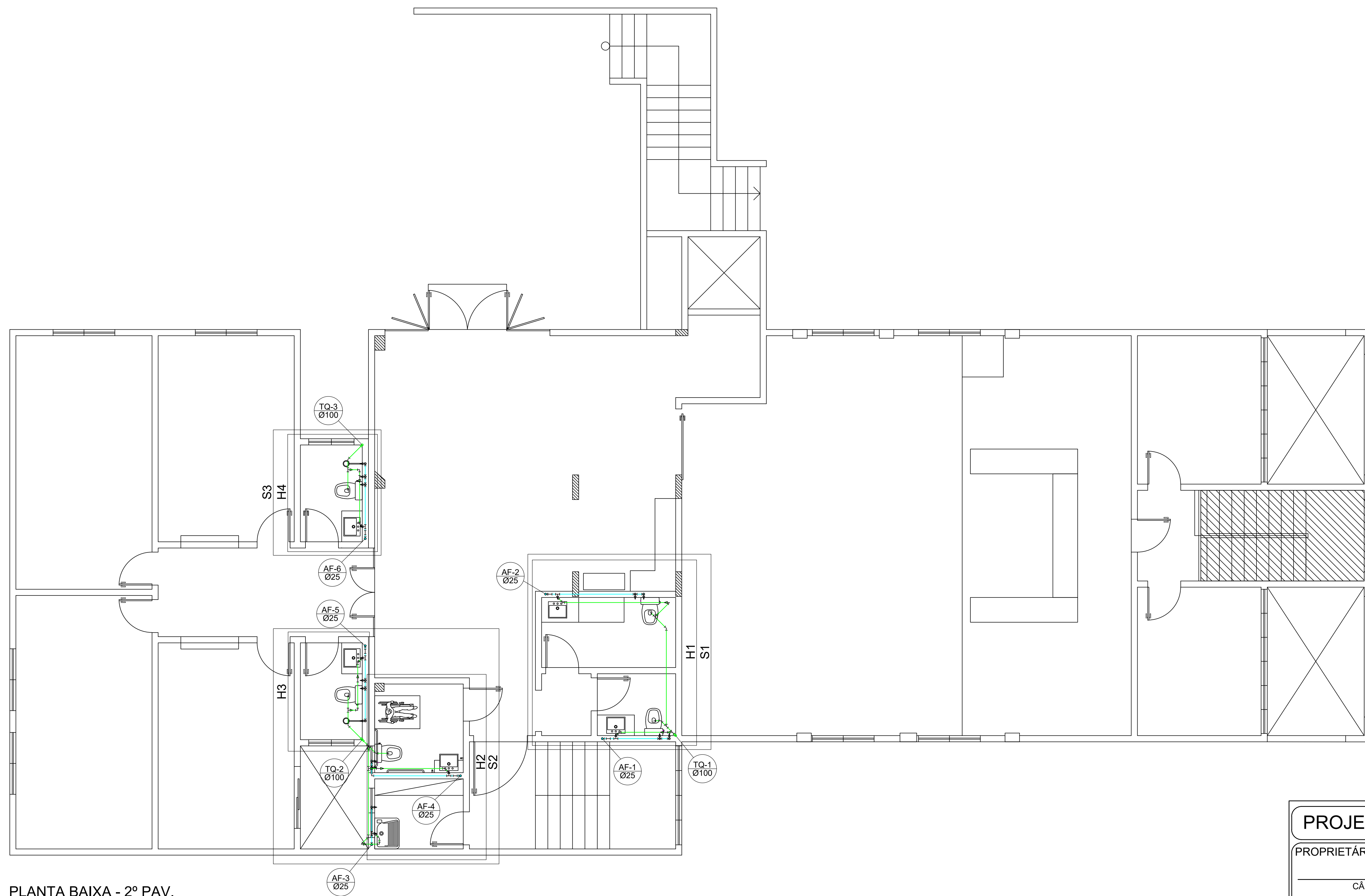
PLANTA BAIXA - 2º PAV. ESCALA: 1/50
